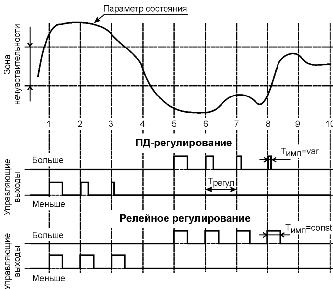
Рис. 1 – Формирование управляющего воздействия для различных регуляторов
