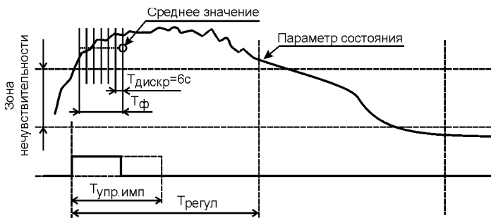
Рис. 25 – Соотношения между временными параметрами регулятора
