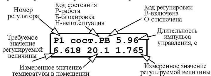
Рис. 28 – Экран состояния регулятора типа 1
